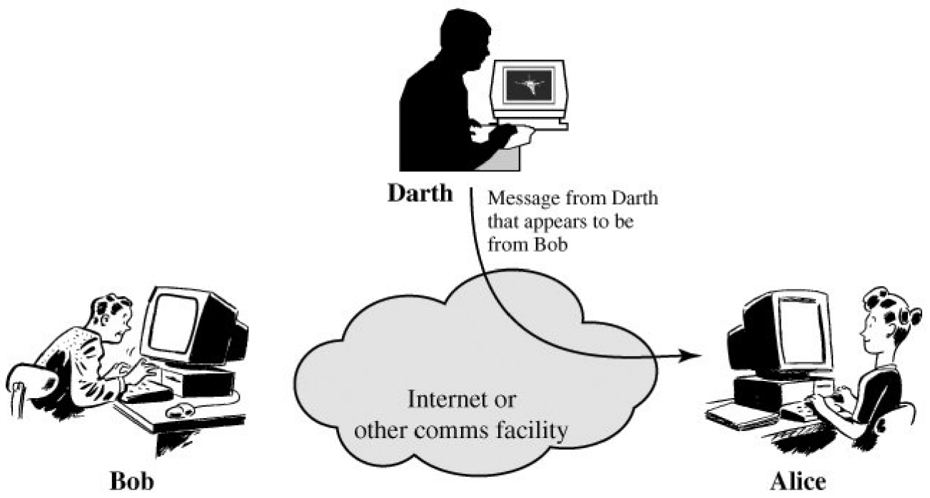
(a) Masquerade
