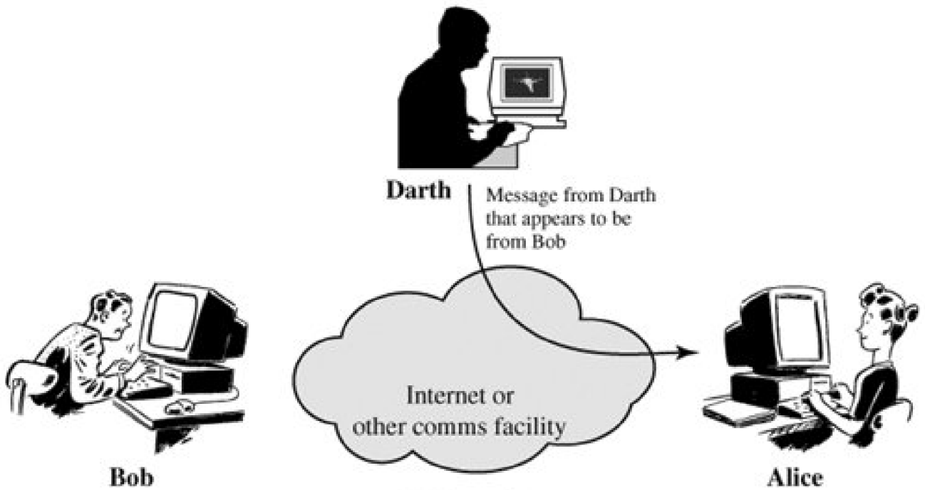
(a) Masquerade
